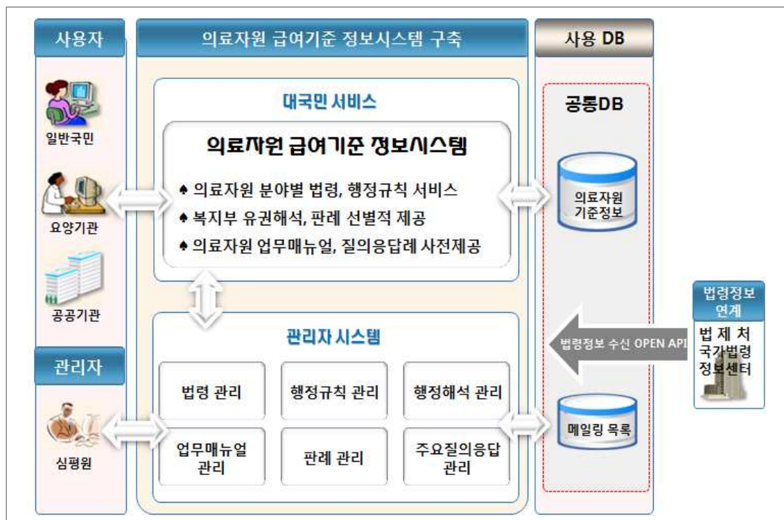
【그림2】 시스템 구성도
